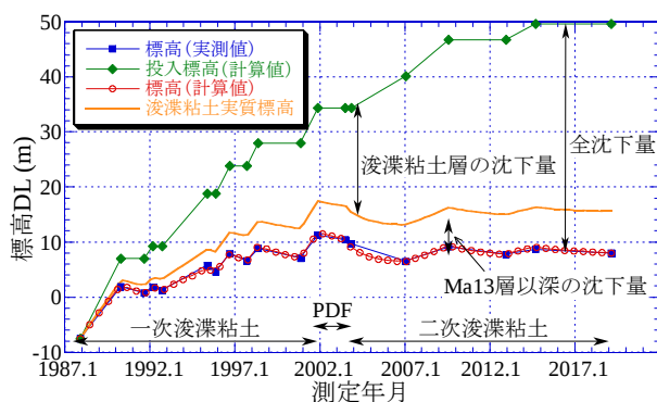
図8 測点3-6での泥面標高の経時変化
