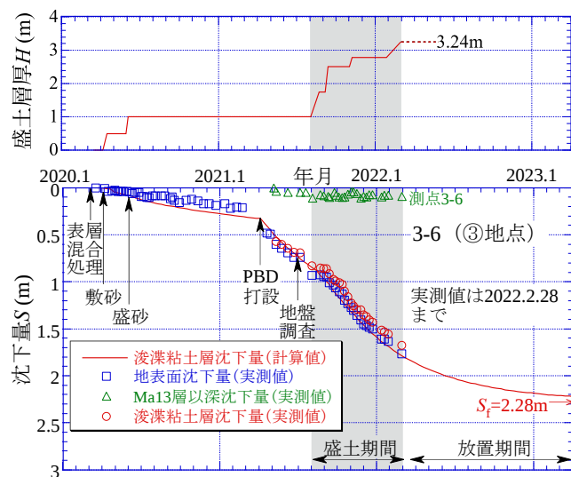
図 10 測点 3-6 での圧密曲線と盛土の経時変化
