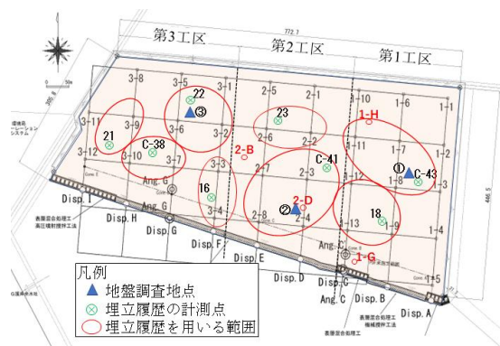
図6 浚渫粘土層の泥面標高測点
