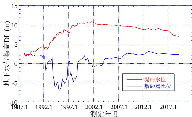
図4 夢洲2区内の堤内水位と敷砂層水位の測定結果
