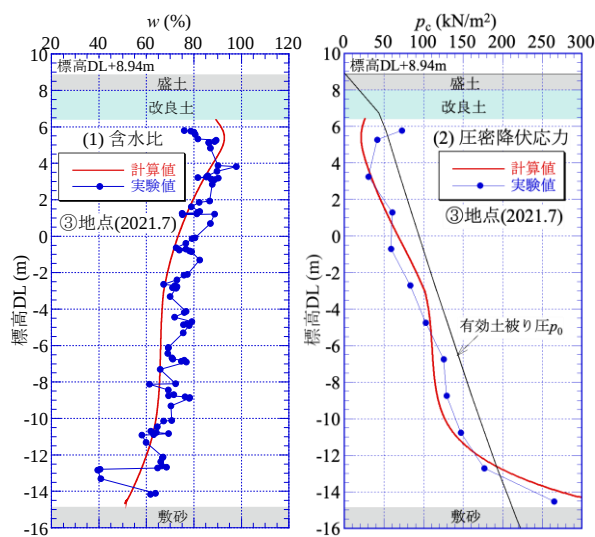
図 11 2021 年 7 月時点の w_n , p の実測値と計算値の比較
