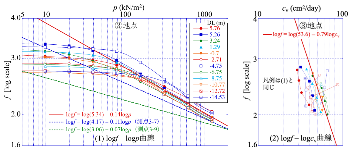
図3 夢洲2区③地点の浚渫粘土層の圧縮曲線( \log f - \log p 曲線)と圧密係数 c_v ( \log f - \log c_v 曲線)
