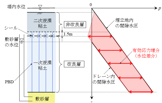
図5 PBD 打設状態と有効応力増分の模式図
