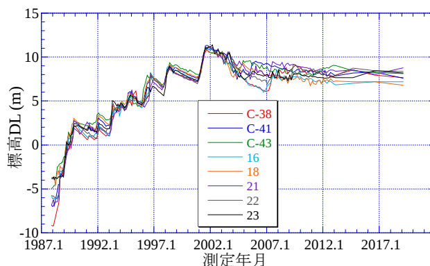
図7 2区内の浚渫粘土層の泥面標高の経時変化
