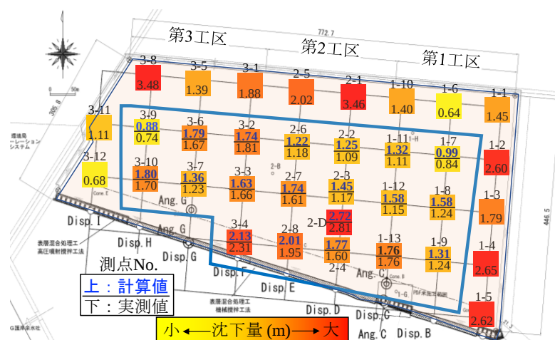
図1.2 2022年2月28日時点の沈下量
