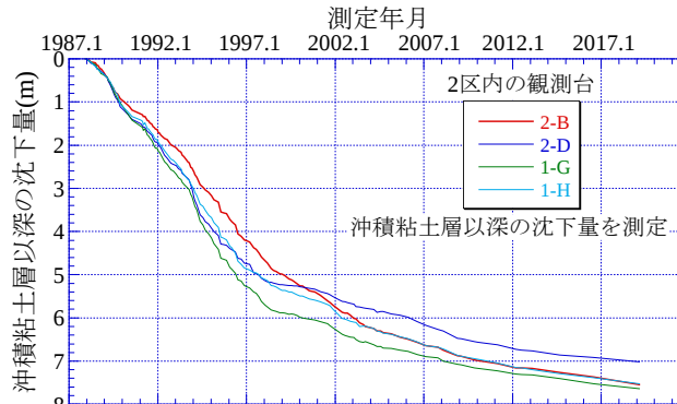
図9 2区内の沖積粘土層以深の圧密曲線
