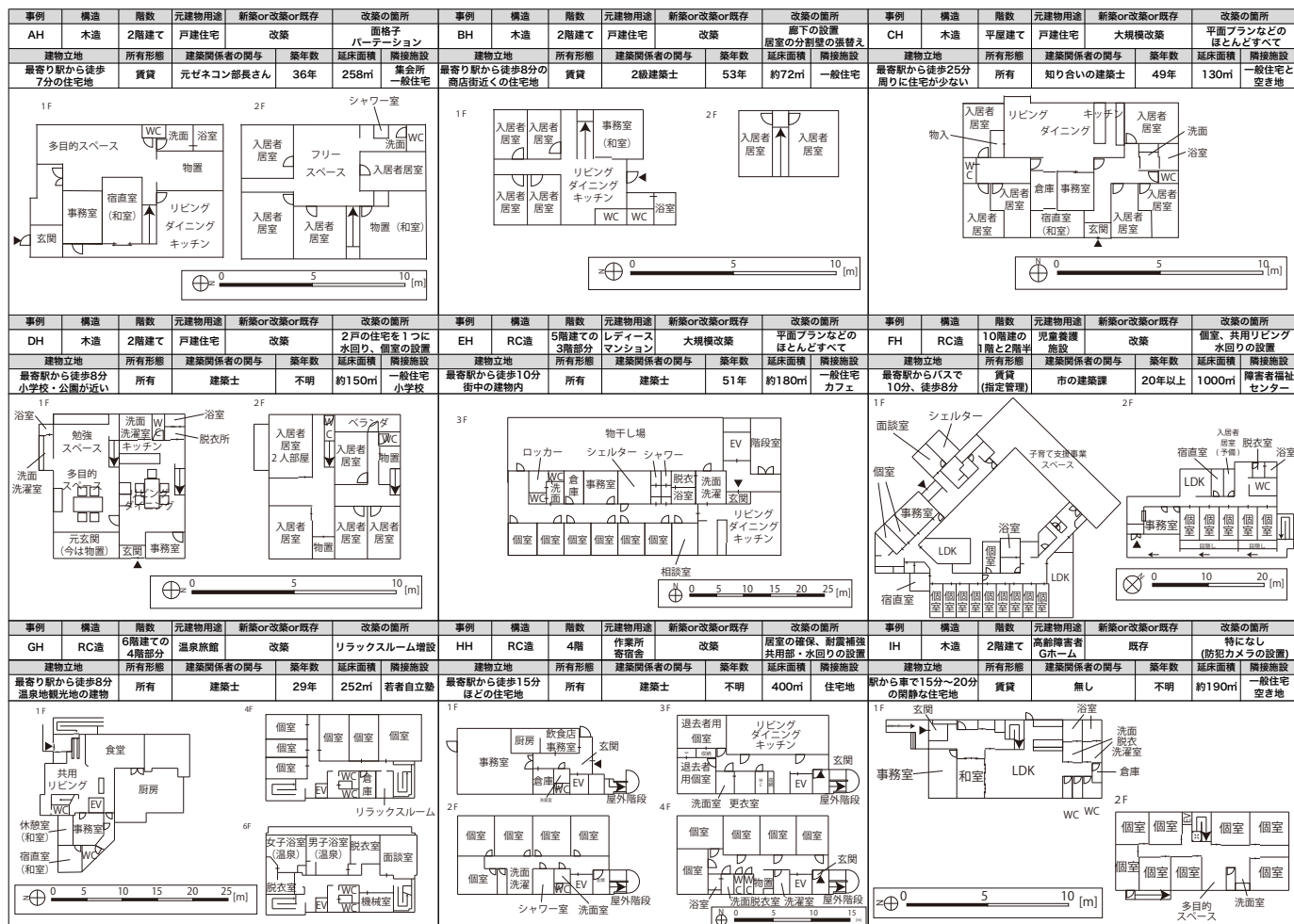
図3 事例9事例平面図
